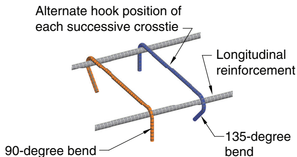
Fig. R25.3.5—Crosstie.
